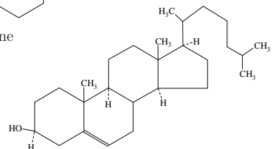
Cholestérol
