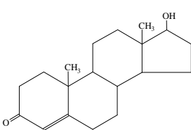
Testostérone
